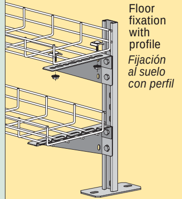
Wall fixation Fijación a la pared
