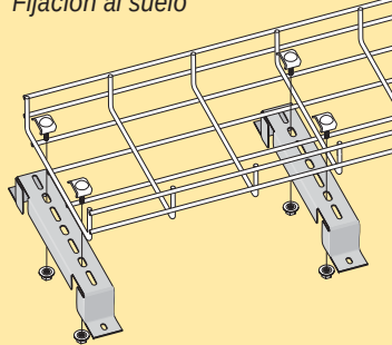
Floor fixation Fijación al suelo
