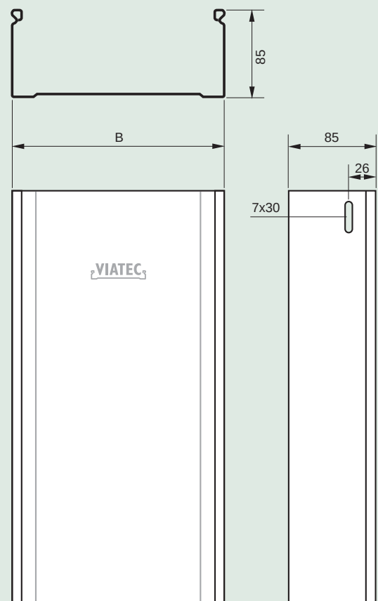
Cable tray section* Sección bandeja*
