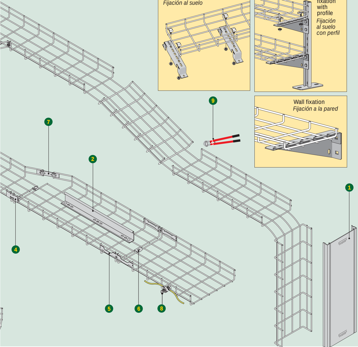
Floor fixation Fijación al suelo
